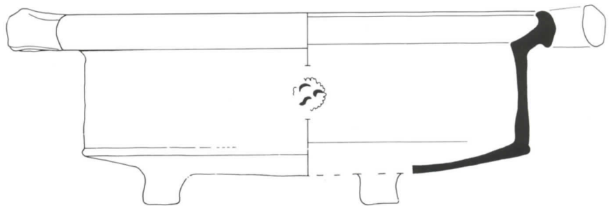
Afb. 44. Kookpan met het merk met de drie halve manen (Stichting Stadsarcheologie Nijmegen); tekening J. R. A. M. Thijssen.
